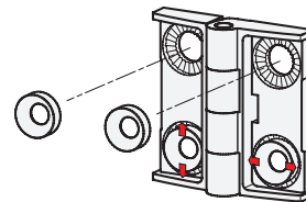
Funktionsprinzip (Form BJ)
