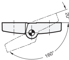
Schwenkbereich
